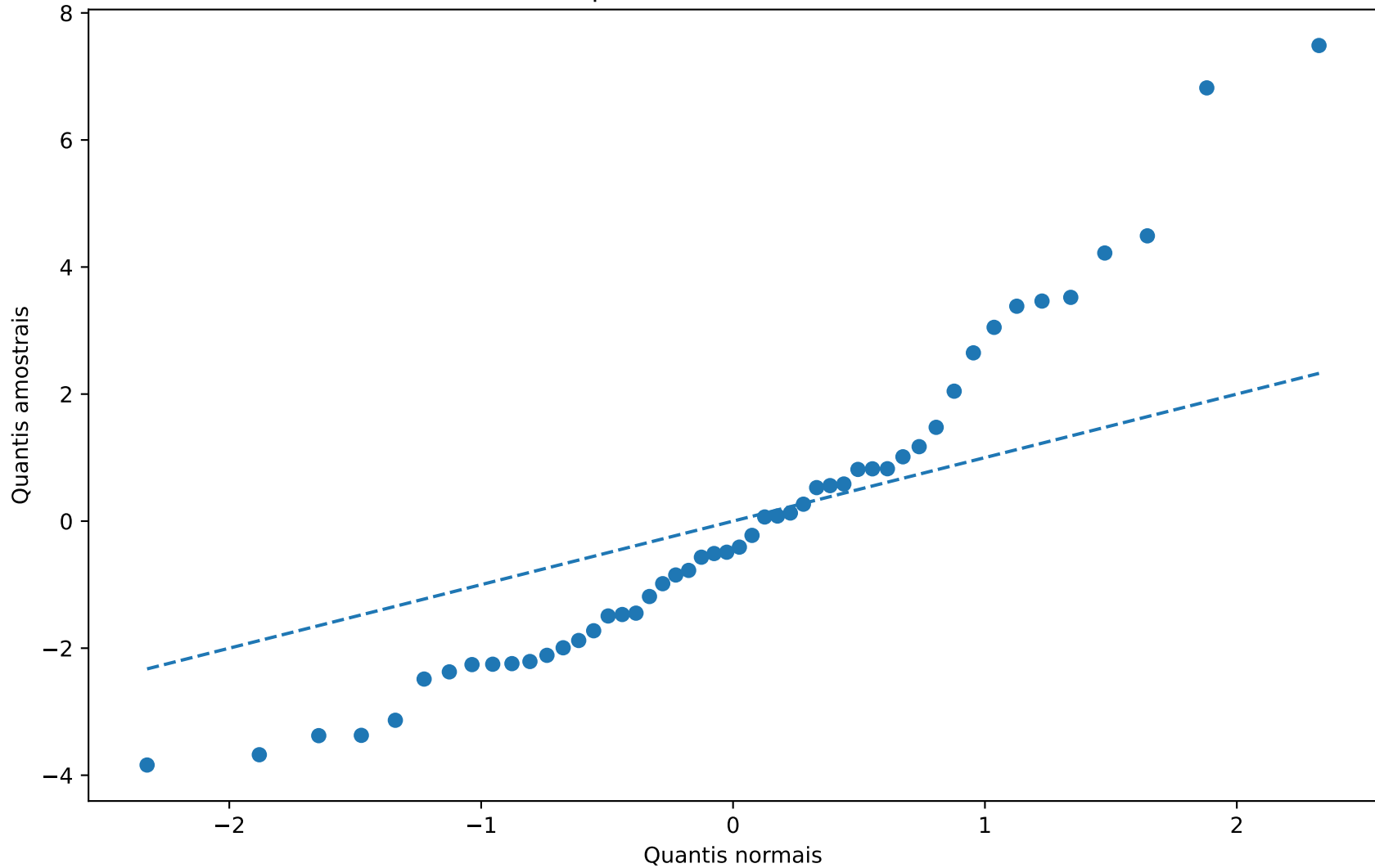
QQ plot do resíduo estrutural
